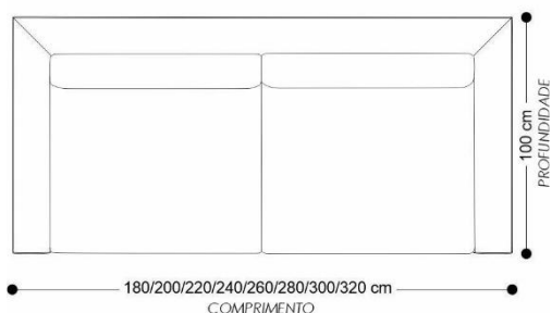
MÓDULO FIXO DOIS BRAÇOS
